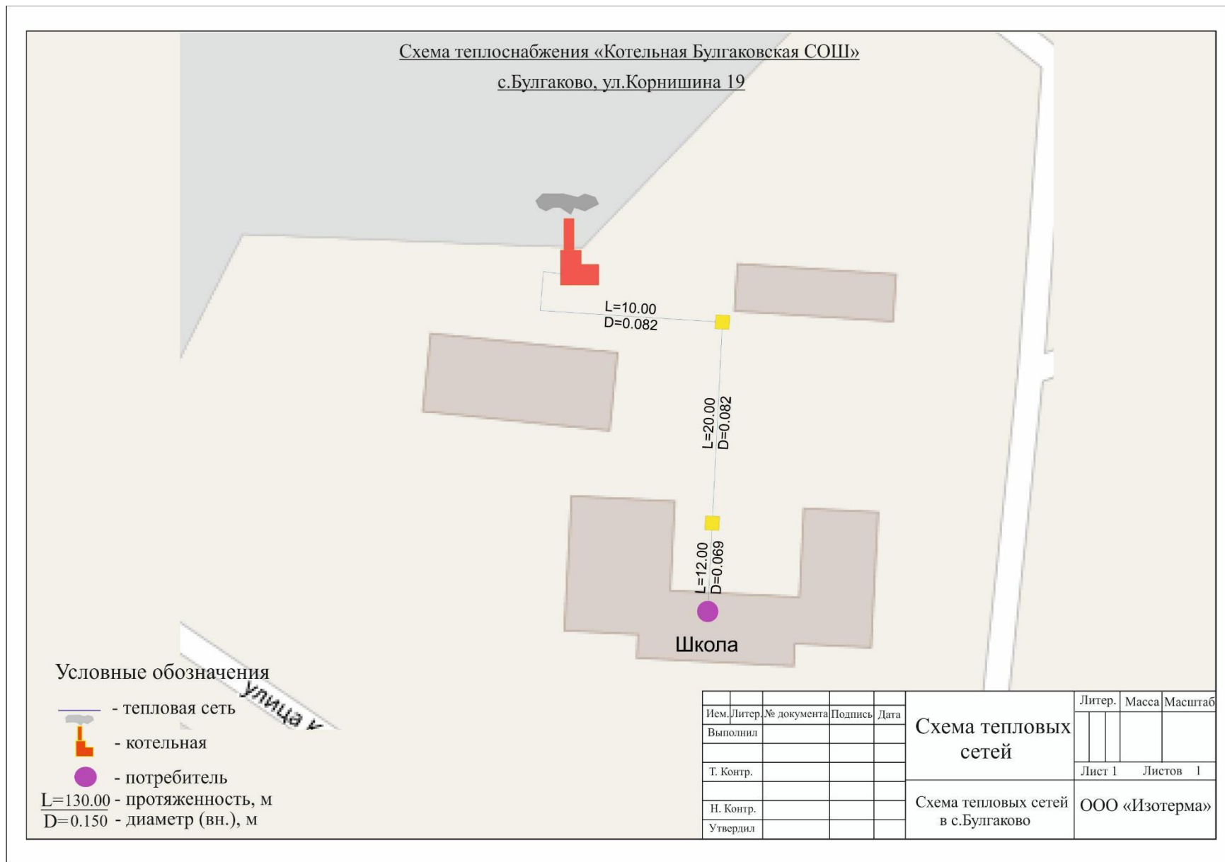
Рисунок 1. Зона действия котельной Булгаковская СОШ
